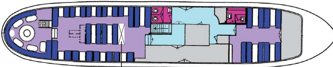
PÄÄKANSI MAIN DECK
