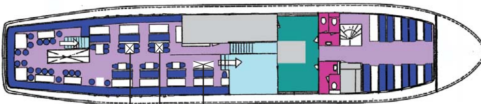
PÄÄKANSI MAIN DECK
